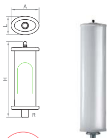
Manguito dieléctrico
