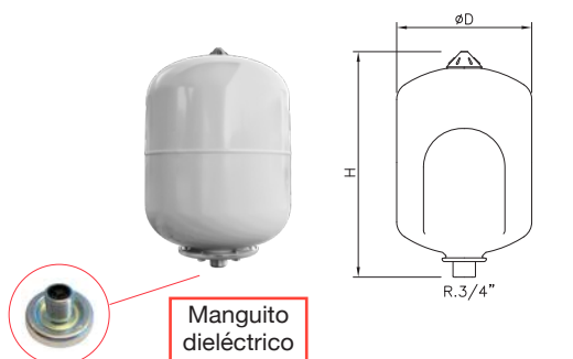
Manguito dieléctrico
