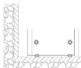
Installation horizontale sur les supports
