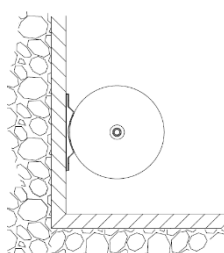
Installation horizontale en utilisant des supports
