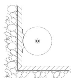
Installation horizontale en utilisant des supports
